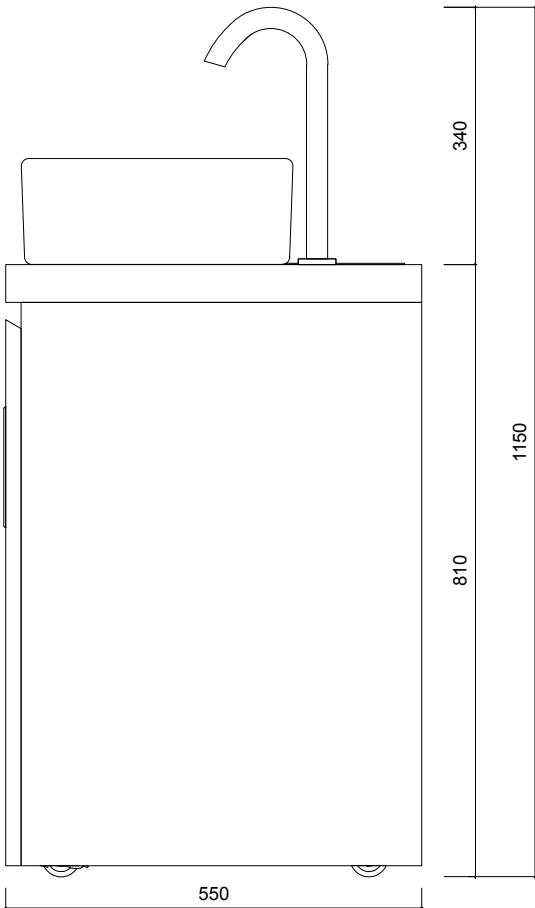
側面
