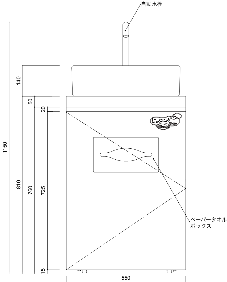
正面
